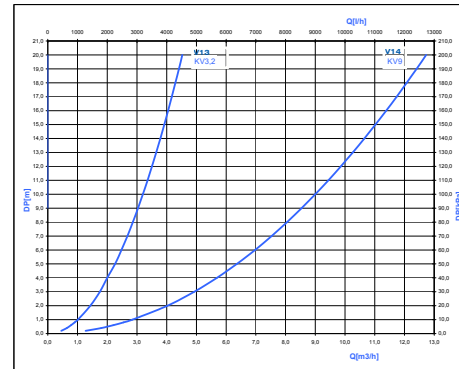
Grafico Portata Flow rate diagram Debit Durchflußdiagramm
